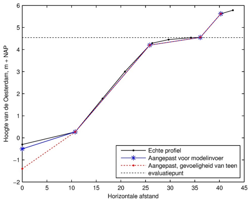
Figuur 2.5 Aanpassing aan de schematisatie van het Oesterdam profiel ten behoeve van de graserosieberekeningen.
